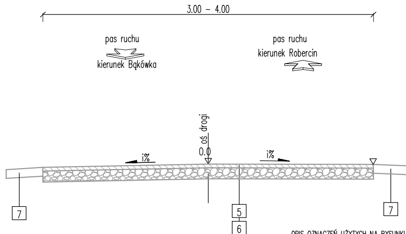
Przekrój normalny – ul. Kolonia w Woli Gołkowskiej – stan istniejący
