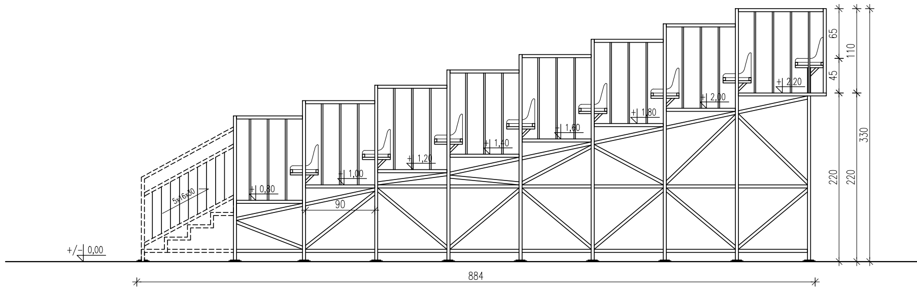
Przekrój—skala 1:50 Rysunek poglądowy trybuny stelażowej. Stadion Miejski w Piasecznie.
