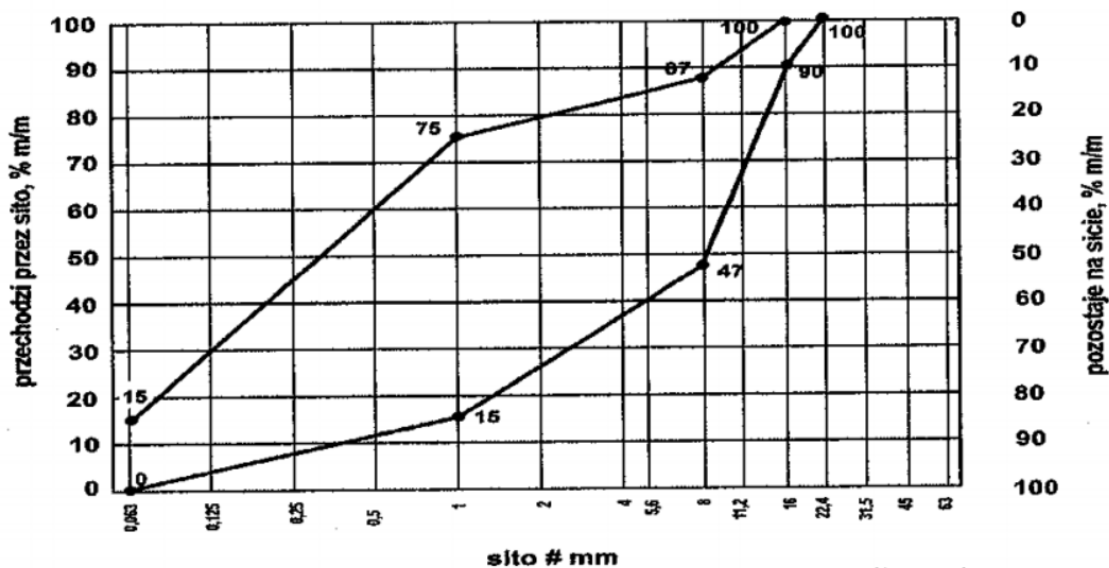
Rys. 4. Mieszanka kruszyw 0/16 do górnej warstwy podłoża ulepszonego
