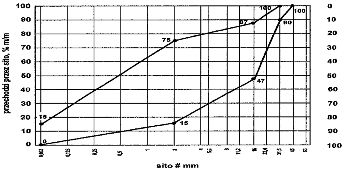
Rys. WT-4. Mieszanka niezwiązana 0/31,5 do nawierzchni z kruszywa niezwiązanego.
