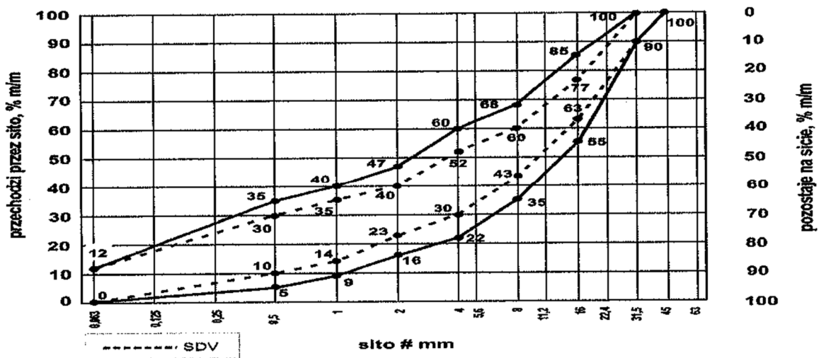
Rys. WT-4. Mieszanka niezwiązana 0/31,5 do górnej warstwy podbudowy pomocniczej.
