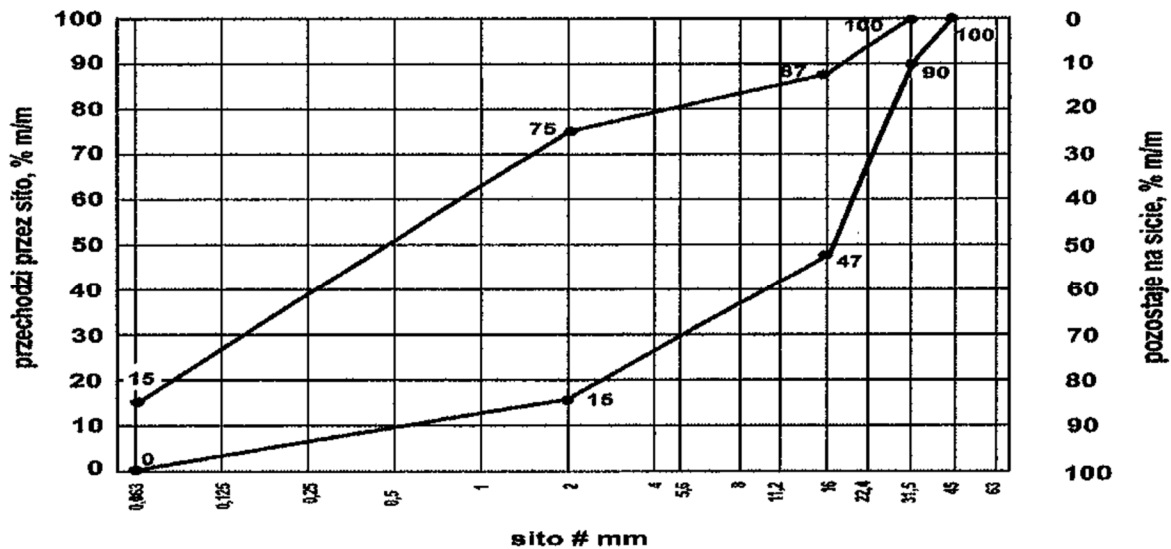
Rys. WT-4. Mieszanka niezwiązana 0/31,5 do nawierzchni z kruszywa niezwiązanego.
