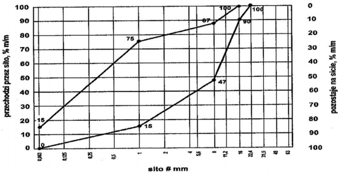
Rys. 4. Mieszanka kruszyw 0/16 do górnej warstwy podłoża ulepszanego
