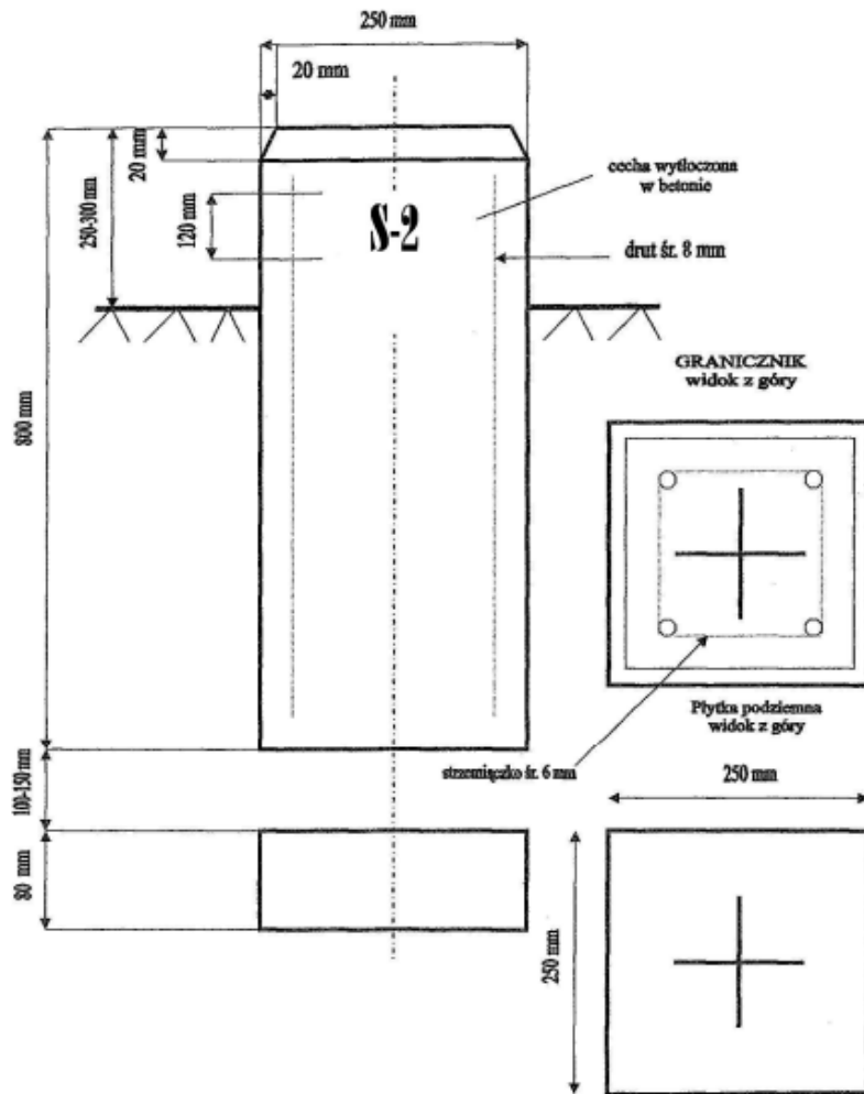
Rys. 2. Betonowy punkt graniczny z cechą np. „S-2”
