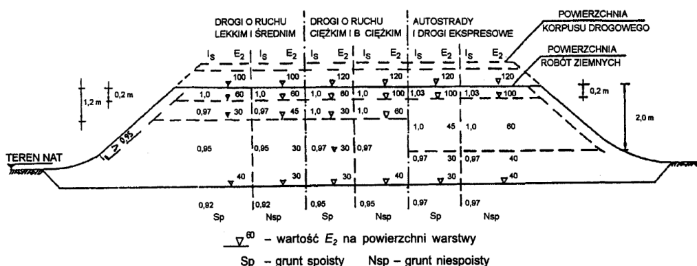
Rysunek 3 – Wartości wymagane w nasypach: wskaźnika zagęszczenia I_s i wtórnego modułu odkształcenia E_2 , megapaskal
