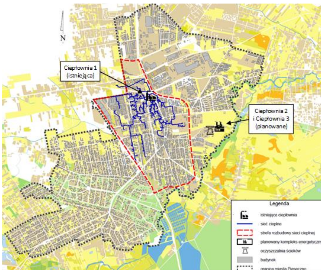
System ciepłowniczy w Piasecznie
