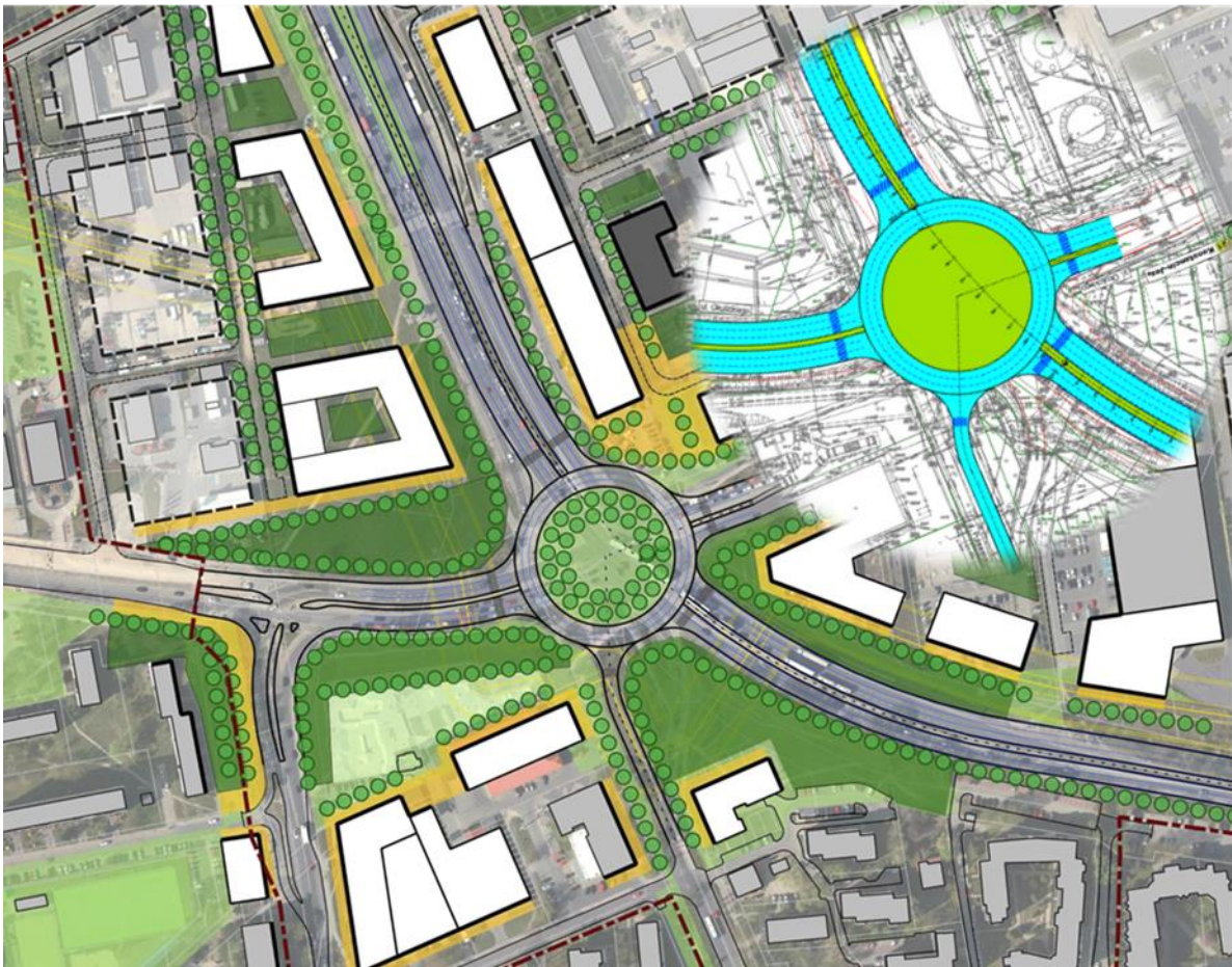
Koncepcja urbanistyczna i drogowa rozwiązania skrzyżowania z ul. Okulickiego zlecona przez UMIG
