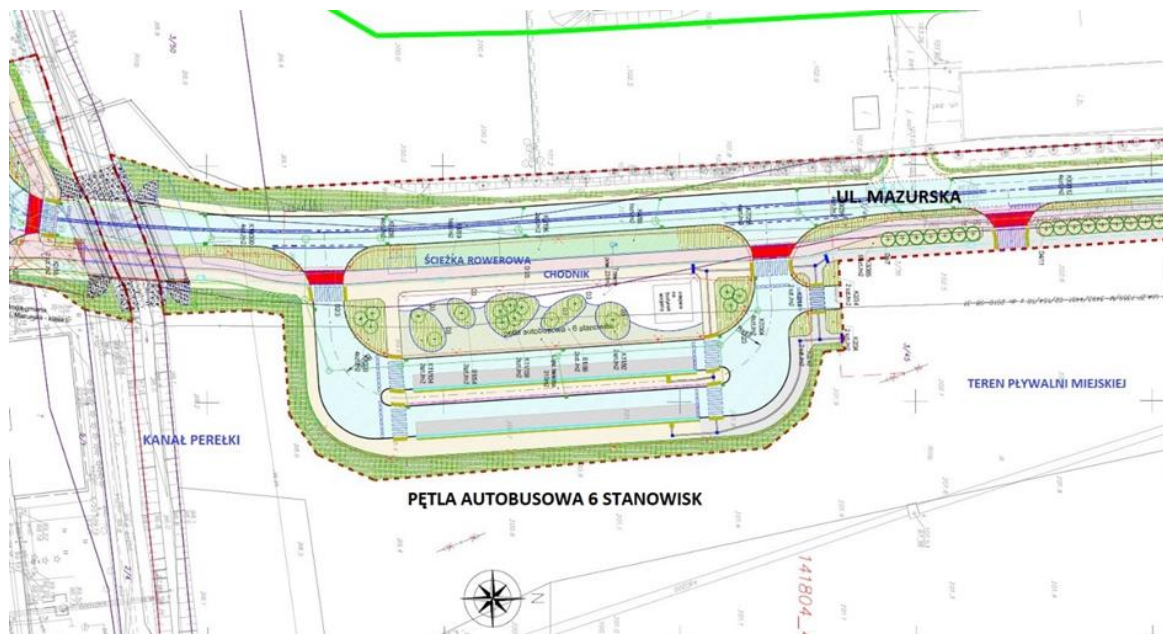
Rysunek 2 Pętla autobusowa w ciągu drogi ul. Mazurskiej w Piasecznie
