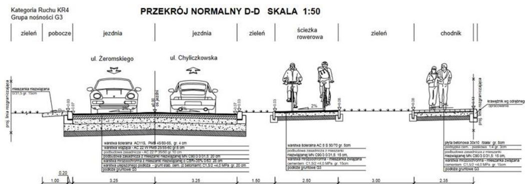
Rysunek 1 Przekrój poprzeczny projektowanej ul. Mazurskiej na wysokości planowanej miejskiej pływalni
